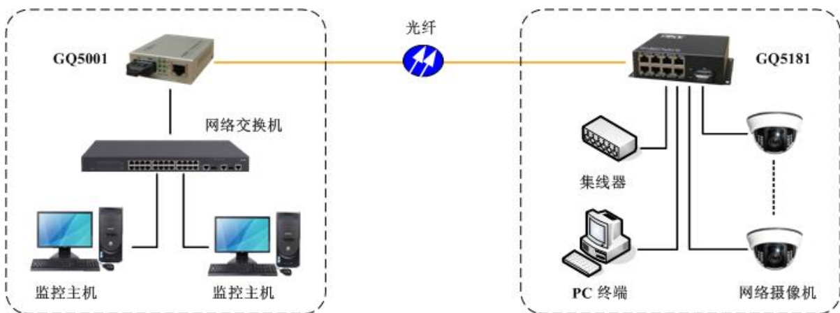
方案一：光纤点对点组网
